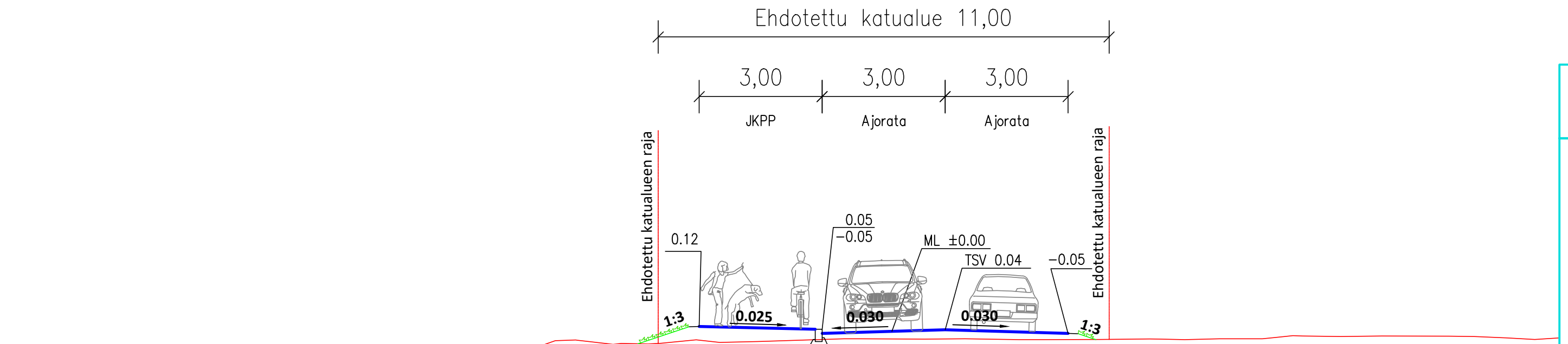
MUSTIMÄENTIE TYYPPIPOIKKILEIKKAUS 1:100 PL 150
