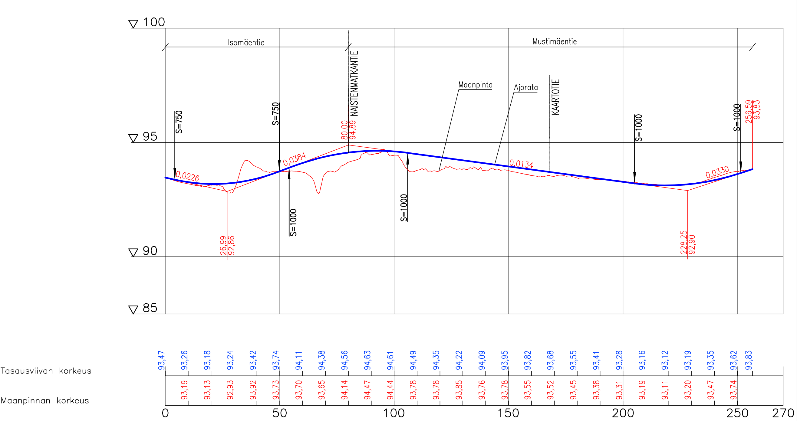
Isomäentie plv 0–81, Mustimäentie plv 81–256 pituusleikkaus 1:1000/1:100
