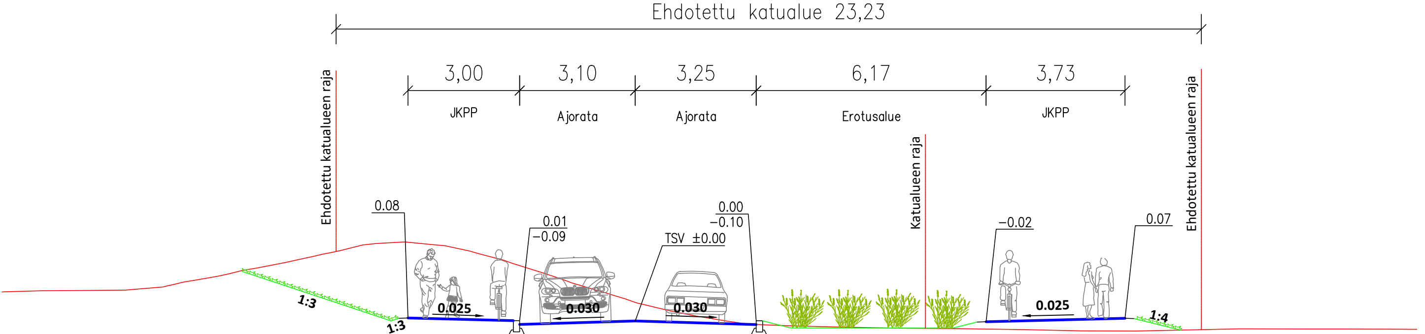
ISOMÄENTIE TYYPPIPOIKKILEIKKAUS 1:100 PL 40
