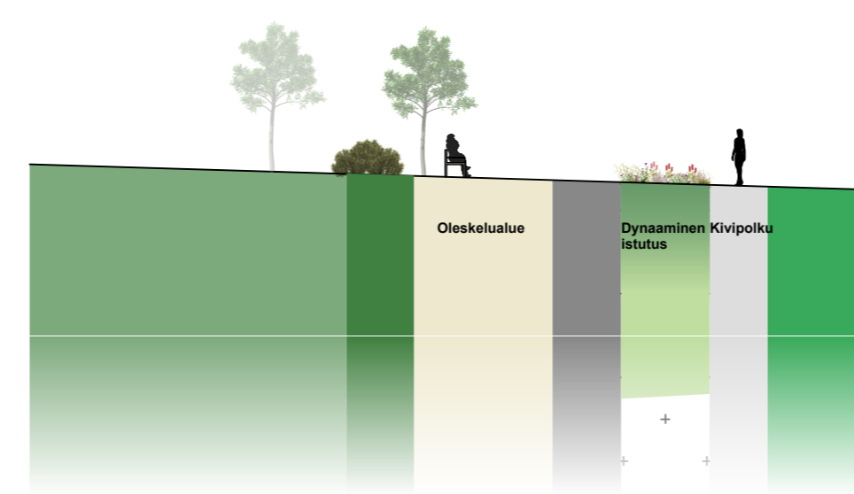
Poikkileikkaus A-A 1:200
